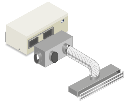
Kit gainable avec émission sur diffuseurs linéaires Kanalisation mit Ausgabe über linearen Diffusoren
