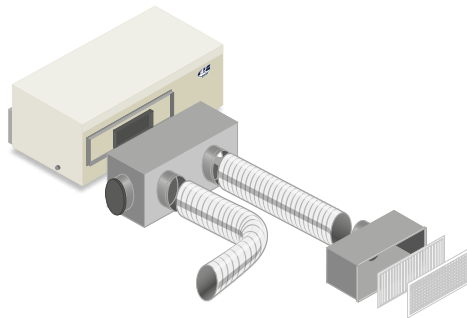
Kit gainable vers 2-3-4 sorties Kann an 2-3-4 Ausgänge geleitet werden
