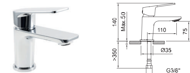
Lavabo monomando con aireador y flexibles 3/8" >350mm. Single-lever basin mixer with aerator and flexible hoses 3/8" >350mm. Mitigreur lavabo avec aérateur et flexibles de raccordement 3/8" >350mm.
