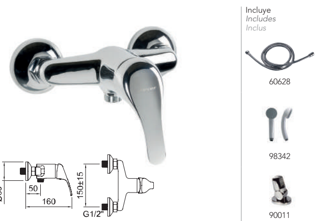
Ducha monomando. Single-lever shower mixer. Mitigeur douche.
