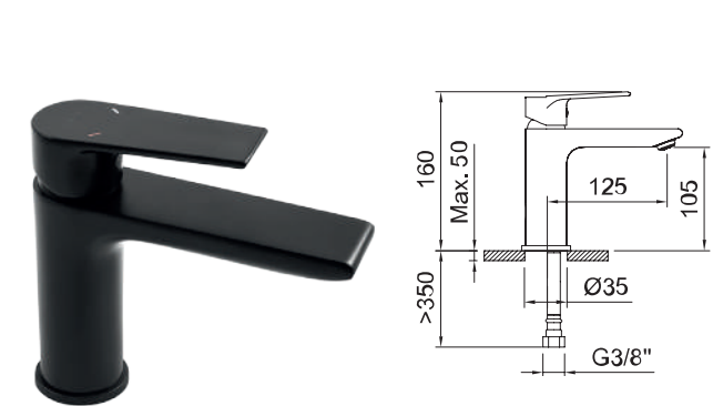
LAVABO 105 Basin mixer 105 Mitigeur lavabo 105
