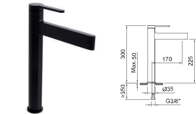
Lavabo alto monomando con aireador y flexibles 3/8" >350mm. Single-lever tall basin mixer with aerator and flexible hoses 3/8" >350mm. Mitigeur lavabo haut avec aérateur et flexibles de raccordement 3/8" >350mm.
