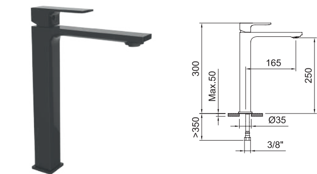
LAVABO 250 Basin mixer 250 Mitigeur lavabo 250
