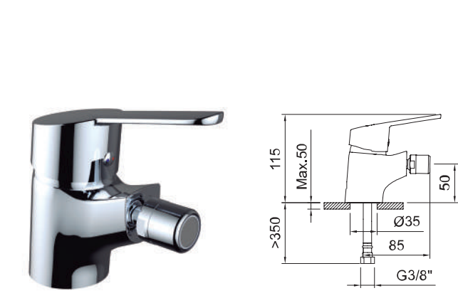
BIDÉ 50 Bidet mixer 50 Mitigeur bidet 50
