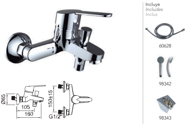
Baño-ducha monomando con aireador e inversor automático. Single-lever bath-shower mixer with aerator and automatic diverter. Mitigeur bain-douche avec aérateur et inverseur automatique.
