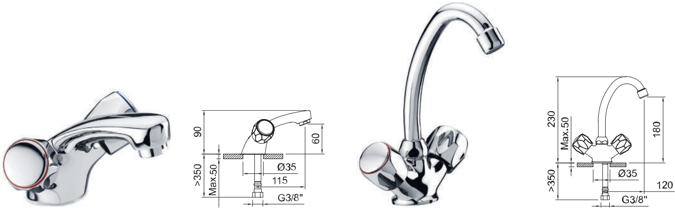
Lavabo bimando con aireador y flexibles 3/8" >350mm. Two-handed basin mixer with aerator and flexible hoses 3/8" >350mm. Mélangeur lavabo avec aérateur et flexibles de raccordement 3/8" >350mm. Lavabo bimando con aireador y flexibles 3/8" >350mm. Two-handed basin mixer with aerator and flexible hoses 3/8" >350mm. Mélangeur lavabo avec aérateur et flexibles de raccordement 3/8" >350mm.
