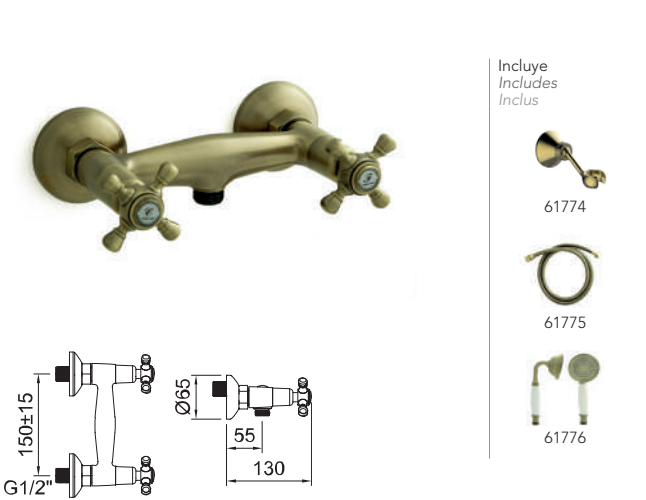
Ducha bimando. Two-handed shower mixer. Mélangeur douche.
