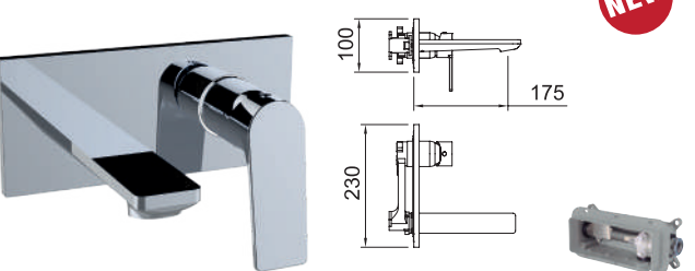
Lavabo empotrar 1/2" con aireador. Concealed basin mixer 1/2" with aerator. Mitigreur lavabo encastré 1/2" avec aérateur.
