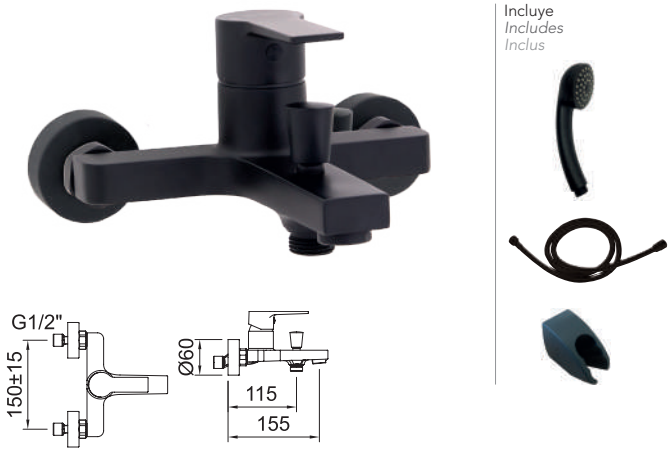
BAÑO-DUCHA Bath-shower mixer Mitigeur bain-douche
