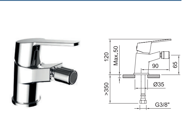
BIDÉ 65 Bidet mixer 65 Mitigeur bidet 65
