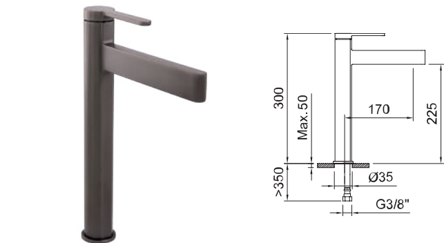
Lavabo alto monomando con aireador y flexibles 3/8" >350mm. Single-lever tall basin mixer with aerator and flexible hoses 3/8" >350mm. Mitigeur lavabo haut avec aérateur et flexibles de raccordement 3/8" >350mm.
