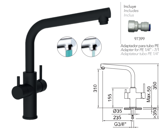
FREGADERO 3 VIAS PARA EQUIPOS DE TRATAMIENTO DEL AGUA 3 way sink mixer for water quality equipment Mitigeur 3 voies pour équipement de traitement de l'eau
