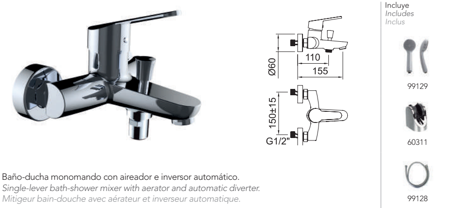
BAÑO-DUCHA Bath-shower mixer Mitigeur bain-douche
