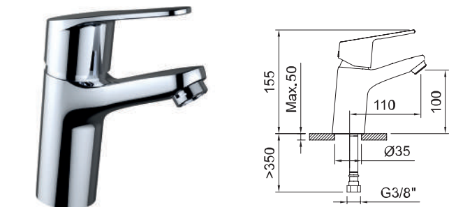
LAVABO 100 Basin mixer 100 Mitigeur lavabo 100
