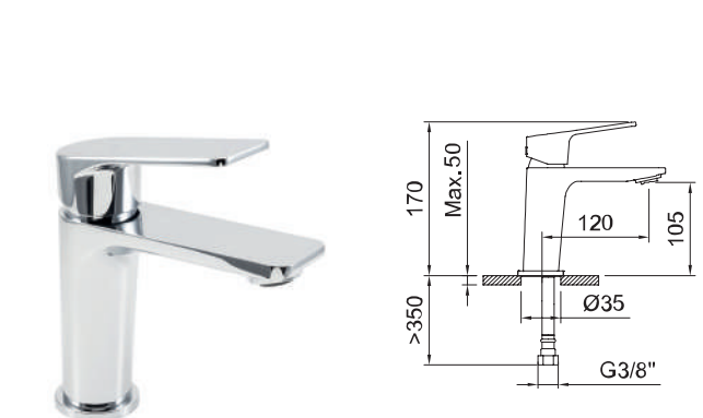
Lavabo monomando con aireador y flexibles 3/8" >350mm. Single-lever basin mixer with aerator and flexible hoses 3/8" >350mm. Mitigreur lavabo avec aérateur et flexibles de raccordement 3/8" >350mm.
