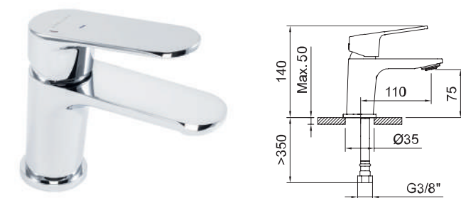
Lavabo monomando con aireador y flexibles 3/8" >350mm. Single-lever basin mixer with aerator and flexible hoses 3/8" >350mm. Mitigeur lavabo avec aérateur et flexibles de raccordement 3/8" >350mm.
