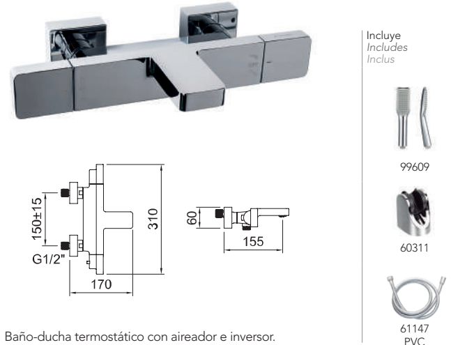
Baño-ducha termostático con aireador e inversor. Thermostatic bath-shower mixer with aerator and diverter. Mitigeur bain-douche thermostatique avec aérateur et inverseur.
