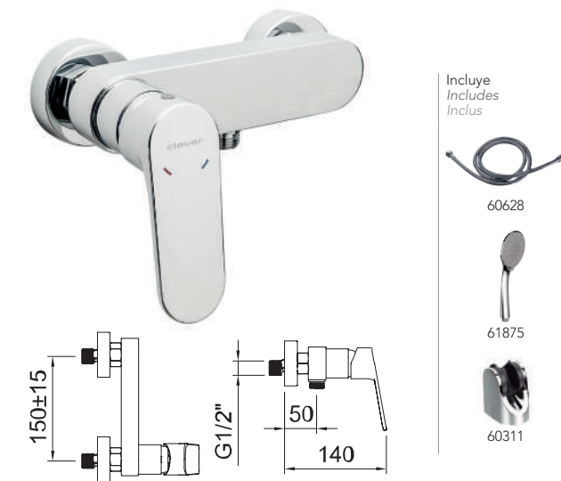
Ducha monomando. Single-lever shower mixer. Mitigeur douche.
