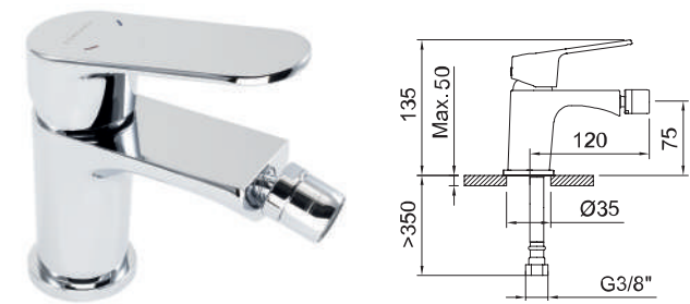
Bidé monomando con aireador a rótula y flexibles 3/8" >350mm. Single-lever bidet mixer with swivel aerator and flexible hoses 3/8" >350mm. Mitigeur bidet avec aérateur rotule et flexibles de raccordement 3/8" >350mm.
