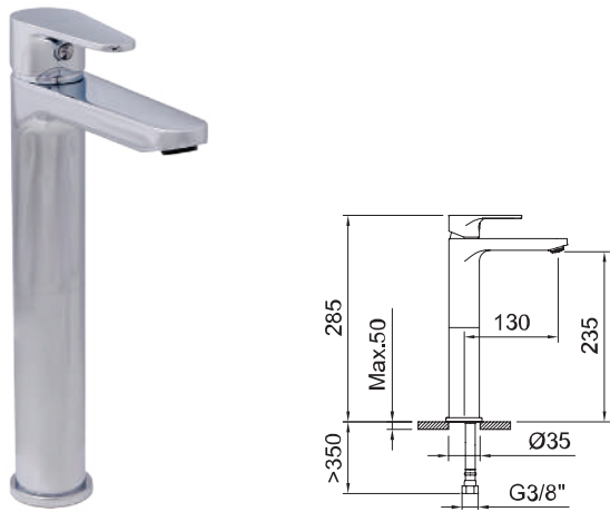
LAVABO 235 Basin mixer 235 Mitigeur lavabo 235
