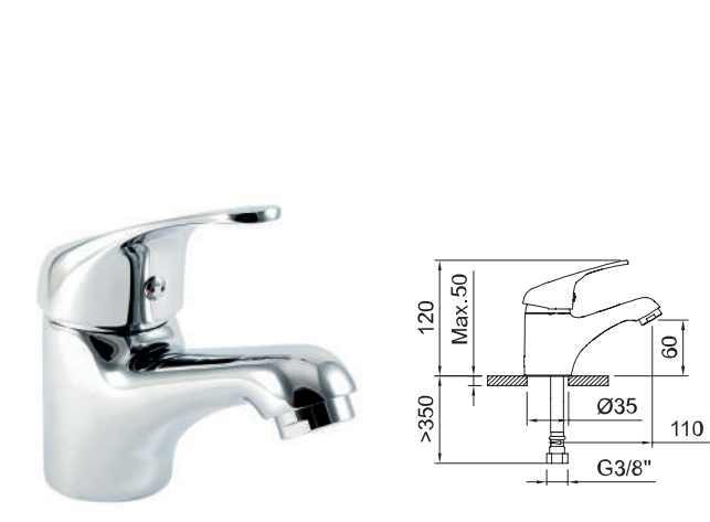
LAVABO 60 Basin mixer 60 Mitigeur lavabo 60
