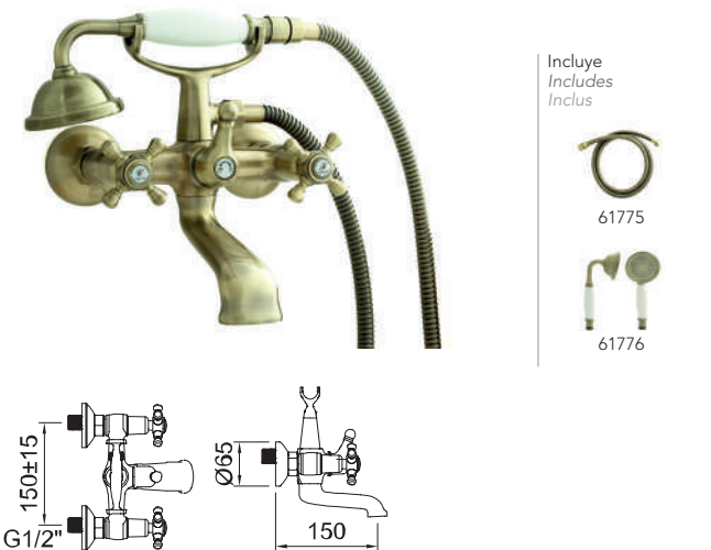
Baño-ducha bimando con inversor. Two-handed bath-shower mixer with diverter. Mélangeur bain-douche avec inverseur.
