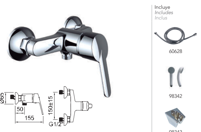
Ducha monomando. Single-lever shower mixer. Mitigeur douche.
