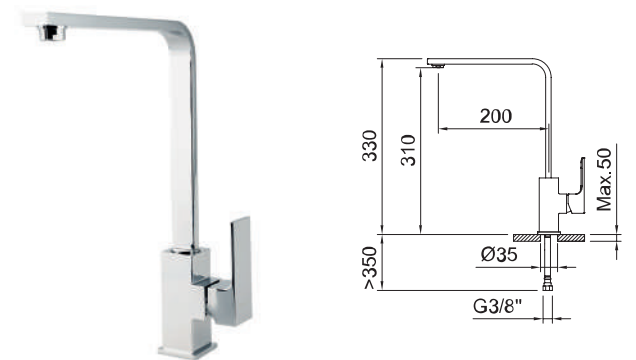
FREGADERO Sink mixer Mitigeur évier
