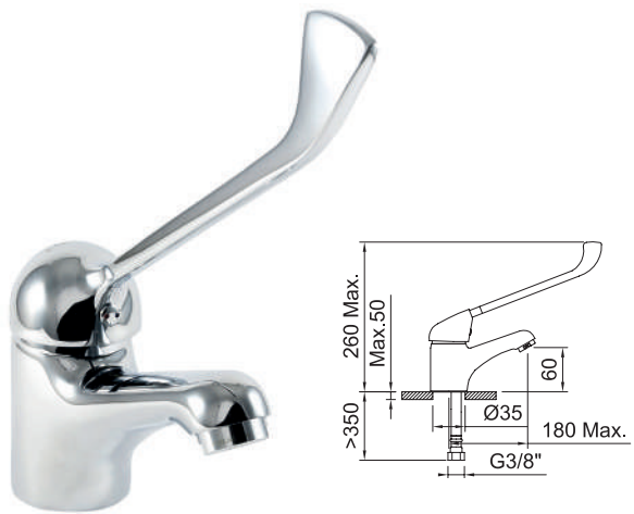
LAVABO CON MANETA GERONTOLÓGICA Basin mixer with medical lever Mitigeur lavabo avec manette médicale
