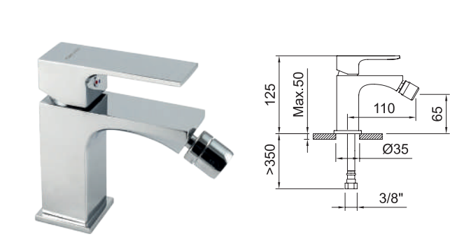
BIDÉ 65 Bidet mixer 65 Mitigeur bidet 65
