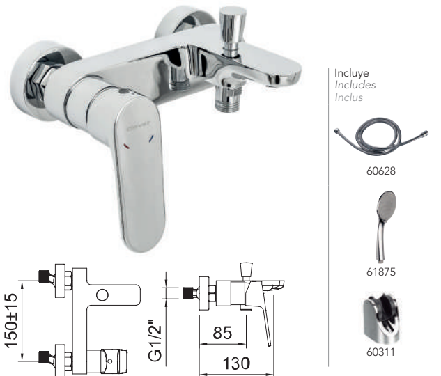
Baño-ducha monomando con aireador e inversor automático. Single-lever bath-shower mixer with aerator and automatic diverter. Mitigeur bain-douche avec aérateur et inverseur automatique.
