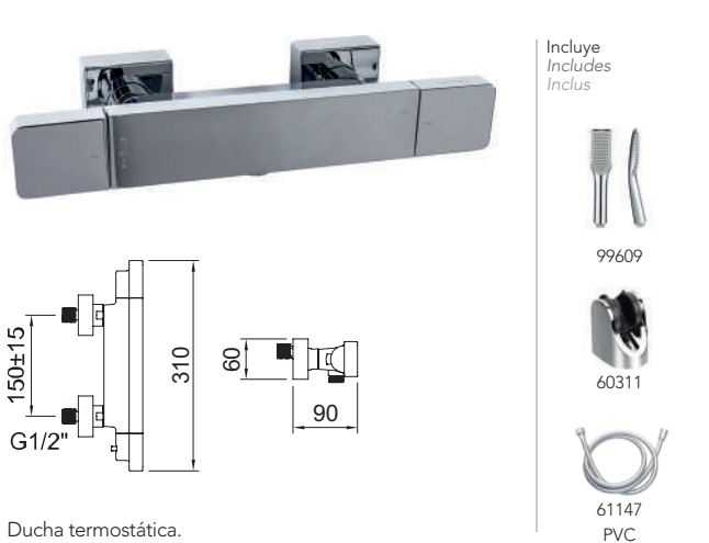
Ducha termostática. Thermostatic shower mixer. Mitigeur douche thermostatique.
