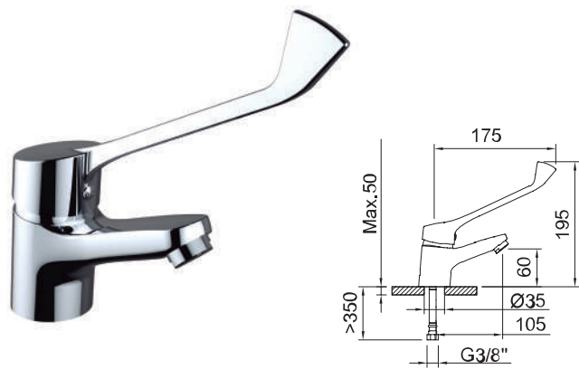
Lavabo monomando con palanca gerontológica, aireador y flexibles 3/8" >350mm. Single-lever basin mixer with medical lever, aerator and flexible hoses 3/8" >350mm. Mitigeur lavabo avec manette médicale, aérateur et flexibles de raccordement 3/8" >350mm.
