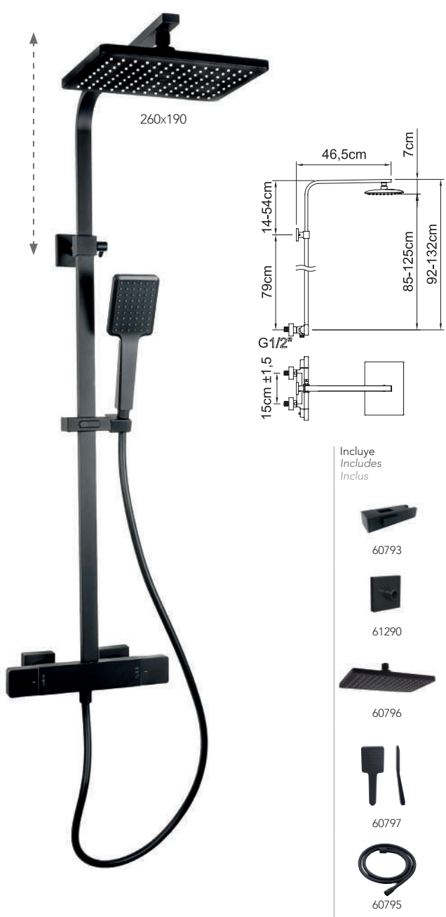
Conjunto de ducha termostática con barra extensible con soporte articulado deslizante. Thermostatic shower set with extendable bar with sliding articulated support. Ensemble de douche thermostatique avec barre extensible avec support articulé coulissant.
