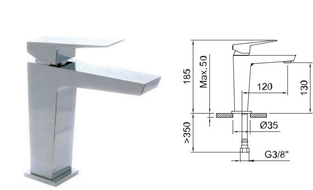
LAVABO 130 Basin mixer 130 Mitigeur lavabo 130
