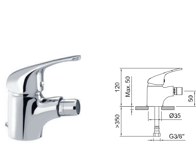
BIDÉ Bidet mixer Mitigeur bidet
