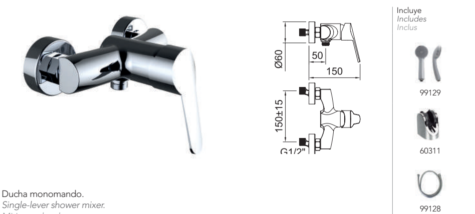
DUCHA Shower mixer Mitigeur douche
