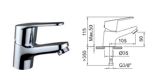
LAVABO 60 Basin mixer 60 Mitigeur lavabo 60
