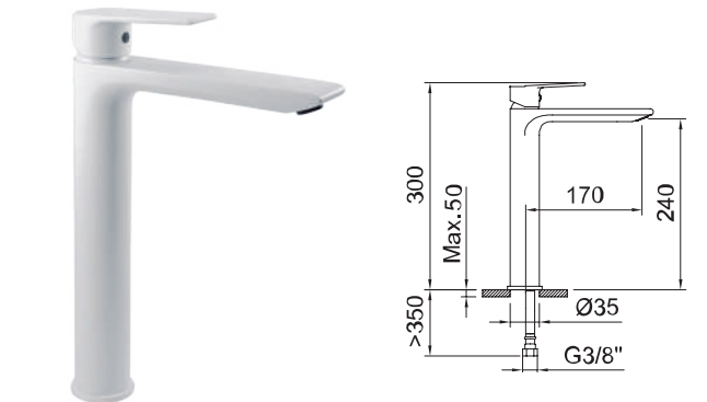
LAVABO 240 Basin mixer 240 Mitigeur lavabo 240
