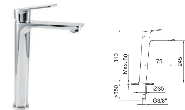
Lavabo alto monomando con aireador y flexibles 3/8" >350mm. Single-lever tall basin mixer with aerator and flexible hoses 3/8" >350mm. Mitigreur lavabo haut avec aérateur et flexibles de raccordement 3/8" >350mm.
