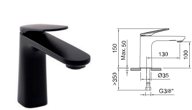
LAVABO 100 Basin mixer 100 Mitigeur lavabo 100
