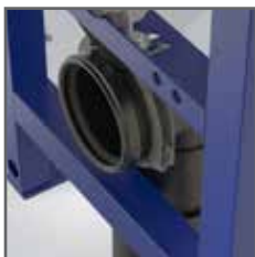
einfach verstellbare Kunststoffschele für Ablaufbogen
