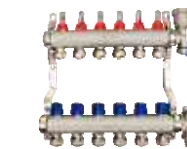
分集水器 Manifold
