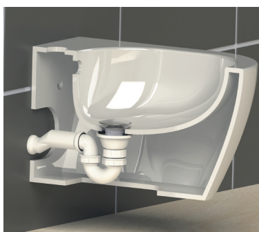
CON ECCENTRICO WITH AN ECCENTRIC PIPE
