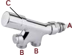
Einrohr Ventilgarnitur für Thermostat- und Handbetätigung mit Sonde. Sonde 315 mm inklusive. Thermostatically controlled single-pipe valve. 315 mm probe included.
