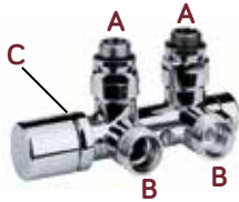
Ventil mit Thermostatanschluss mit by-pass und Rücklaufverschraubung. Ausf. f. Eckmontage Thermostatic angle valve with by-pass and lockshield
