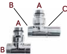
Ventilpaar mit Thermostatanschluss mit Rücklaufverschraubung f. Eckmontage Thermostatic angled valves and lockshield
