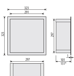
RB 300
