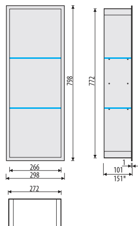
P.PWNP 3080/10 P.PWNP 3080/15*
