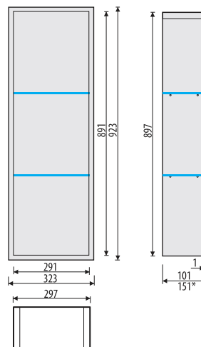
RB 900
