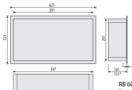
P.PWN 600/10 P.PWN 600/15*
