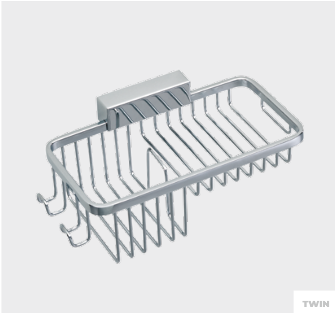
IRIS 2 Duschmittelkorb Wand I420-0000 B= 213 mm, T=116 mm, H=80 mm
