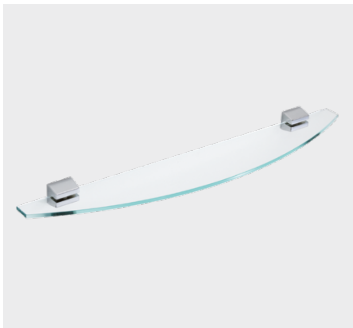
IRIS² Ablage 750 I213-0000 mit Glasplatte 750 mm B=750 mm, T=146 mm, H=46 mm Glasstärke 8 mm
