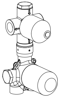
3254MCLT2 P.I. Corpo incasso per miscelatore a 2 vie Concealed body for 2 ways mixer Corps encastrée pour mitigeur 2 vois
