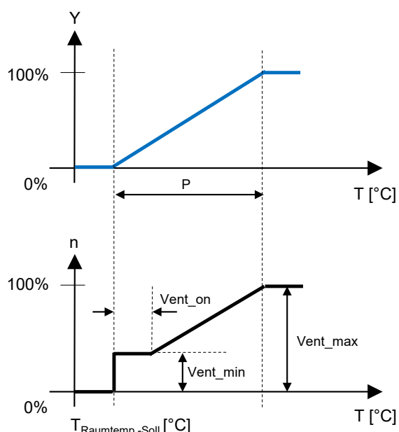
Beispiel Regelungsschema
