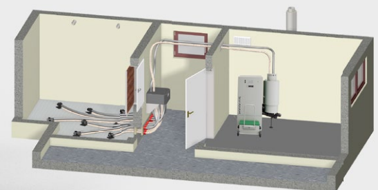
Abbildung: Saugbehälter DIRECT in Kombination mit 8-Punktabsaugung
