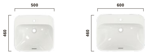
L5615CE Möbelwaschtisch LF 500mm, mit Hahnloch, mit Überlauf Furniture washbasin LF 500mm, with tap hole, with overflow
