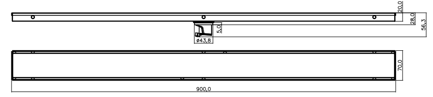
SC9002SP-A 隐形地漏 Size:70*900*1mm 表面处理: 拉丝
