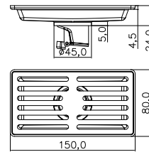
SC1501SP-A 长条地漏 Size:80*150*2mm 表面处理: 拉丝
