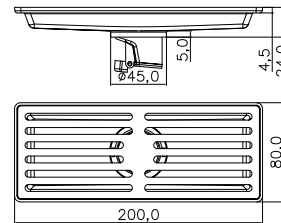
SC2001SP-A 长条地漏 Size:80*200*2mm 表面处理: 拉丝
