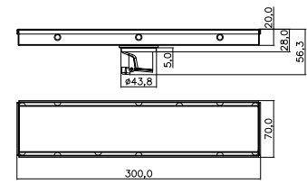
SC3002SP-A 隐形地漏 Size:70*300*1mm 表面处理: 拉丝
