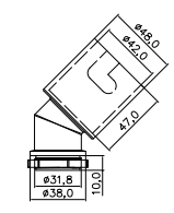
PJ02 洗衣机接头 颜色: 灰色
