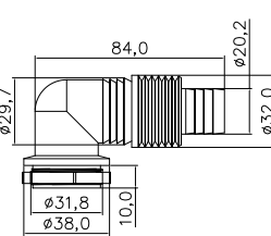
PJ01 洗衣机接头 颜色: 灰色
