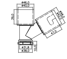
PJ03 洗衣机接头 颜色: 灰色
