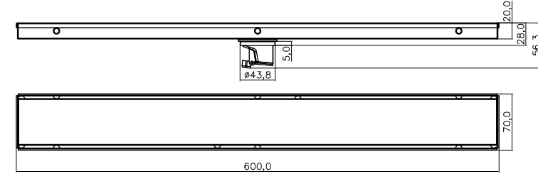
SC6002SP-A 隐形地漏 Size:70*600*1mm 表面处理: 拉丝
