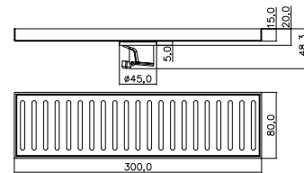
SC3001BA-A 长条地漏 Size:80*300*2mm 表面处理: 哑黑
