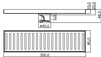
SC3001SP-A 长条地漏 Size:80*300*2mm 表面处理: 拉丝
