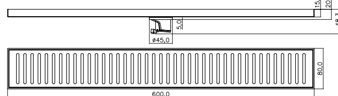
SC6001SP-A 长条地漏 Size:80*600*2mm 表面处理: 拉丝
