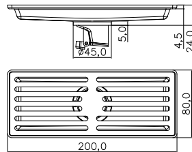
SC2001BA-A 长条地漏 Size:80*200*2mm 表面处理: 哑黑
