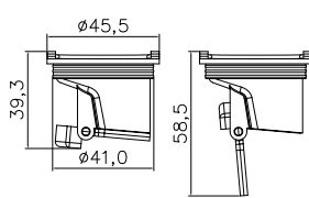
A50 直排地漏芯 颜色: 灰色
