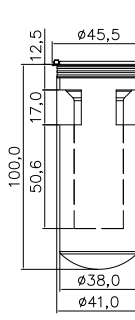
C50PC 水封地漏芯 颜色: 黄铜
