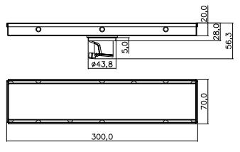
SC3002BA-A 隐形地漏 Size:70*300*1mm 表面处理: 哑黑
