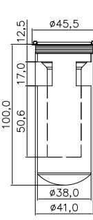
C50SP 水封地漏芯 颜色: 拉丝
