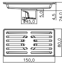
SC1501BA-A 长条地漏 Size:80*150*2mm 表面处理: 哑黑
