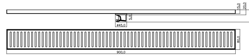
SC9001SP-A 长条地漏 Size:80*900*2mm 表面处理: 拉丝
