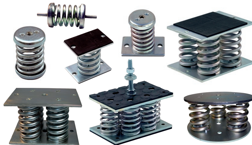
ISOLANTS METALIQUES: Isolateurs à ressort
