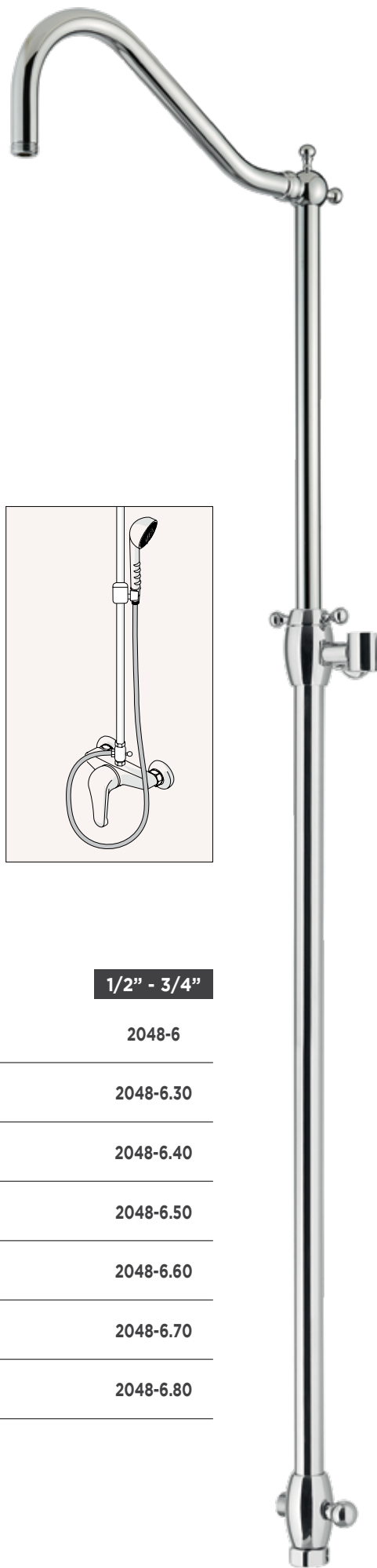
ART. 2048-6 Colonna doccia telescopica ad onda in ottone, regolabile in altezza da 715 a 1135 mm., completa di deviatore per attacco flessibile 1/2"M. Wave telescopic brass shower column, adjustable height from 715 to 1135 mm., diverter with 1/2"M flexible pipe fitting included. Colonne de douche vague télescopique en laiton, hauteur réglable de 715 à 1135 mm., avec inverseur et raccordement de fixation du flexible 1/2"M.
