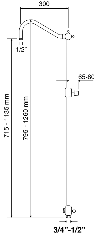
ART. 2048-6 Colonna doccia telescopica ad onda in ottone, regolabile in altezza da 715 a 1135 mm., completa di deviatore per attacco flessibile 1/2"M. Wave telescopic brass shower column, adjustable height from 715 to 1135 mm., diverter with 1/2"M flexible pipe fitting included. Colonne de douche vague télescopique en laiton, hauteur réglable de 715 à 1135 mm., avec inverseur et raccordement de fixation du flexible 1/2"M.
