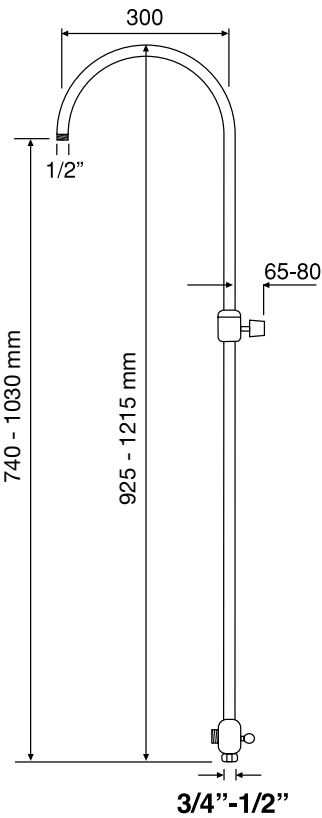
ART. 2051 Colonna doccia telescopica ad arco in ottone, regolabile in altezza da 740 a 1030 mm., completa di deviatore per attacco flessibile 1/2" M. Bow-shaped telescopic brass shower column, adjustable height from 740 to 1030 mm., diverter with 1/2" M flexible pipe fitting included. Colonne de douche télescopique recourbée en laiton, hauteur réglable de 740 à 1030 mm., avec inverseur et raccordement de fixation du flexible 1/2" M.
