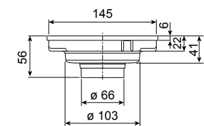
P15/66 uscita/outlet ø 66 mm - ø 103 mm
