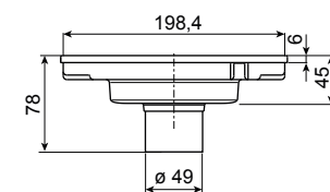
P20/T49 uscita/outlet Ø 49 mm
