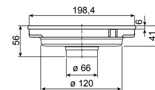
P20/66 uscita/outlet Ø 66 mm - Ø 120 mm
