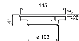
P15/103 uscita/outlet ø 103 mm
