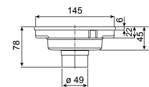
P15/T49 uscita/outlet ø 49 mm
