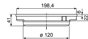
P20/120 uscita/outlet Ø 120 mm
