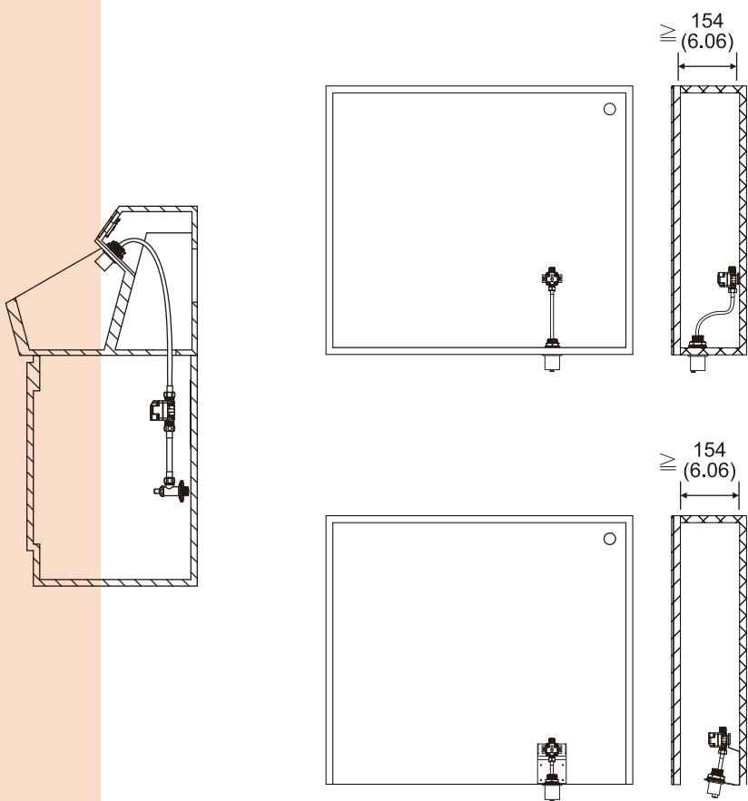
InnoWash FA01 Color : Bright Material : SUS 304 Power : AC
