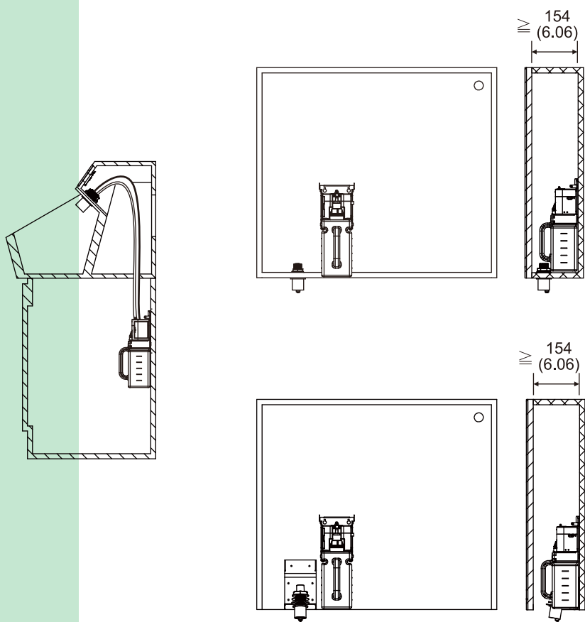
InnoWash SD11 / 21 / 31 Color : Bright Material : SUS 304 Power : AC
