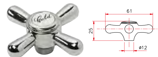
Art. 107 Maniglia Quadrifoglio G.
