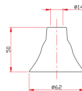
Art. 383 Cappuccio Onda
