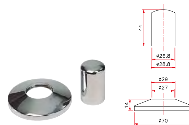
Art. 351 Cappuccio Scorrevole
