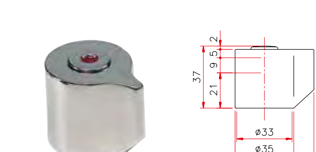
Art. 207 Deviatore Ariete
