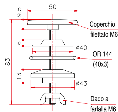
Art.451 Tappo coproforo
