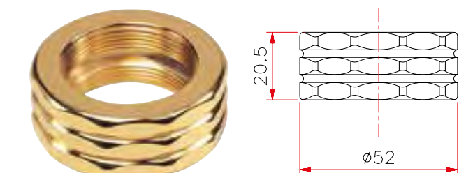
Art. 005 Anello Francia
