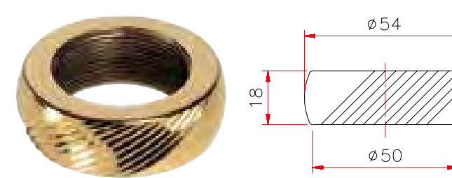
Art. 059 Anello Belgio
