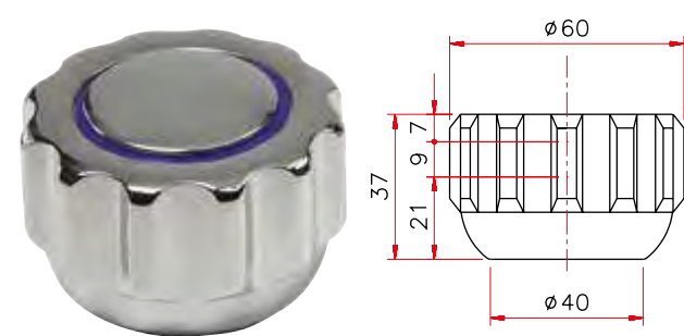
Art. 187 Maniglia Patrizia
