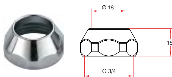
Art.447 Calotta Conica Economica
