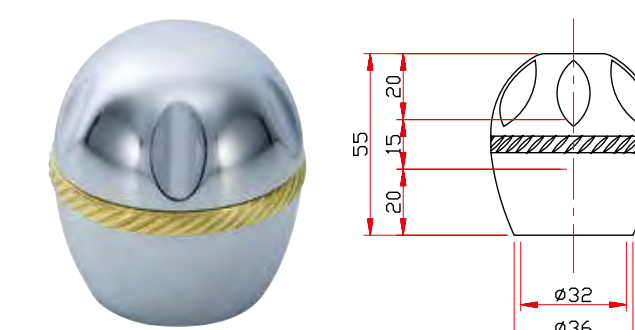
Art. 191 Maniglia Cocò
