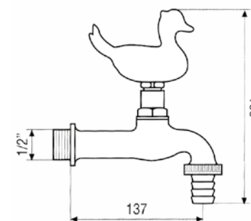
Art. 953 Rubinetto con maniglia anatra Robinet avec poignée à canard Tap with duck handle
