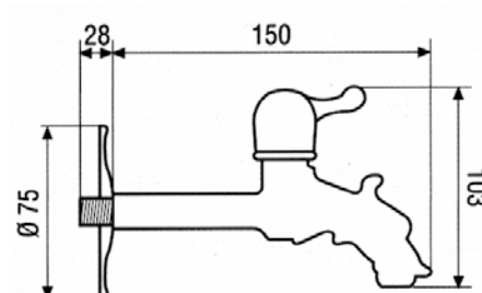
Art. 921 Rubinetto artistico a passo rapido con rosone grande e portagomma Attacco 1/2" M Robinet artistique à pas rapide avec rose grande et porte-tuyau Raccord de 1/2" M Artistic quick pitch tap with big rosette and hose adapte 1/2" M connection
