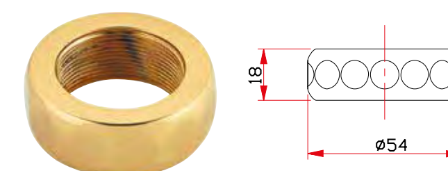
Art. 095 Anello Kenia
