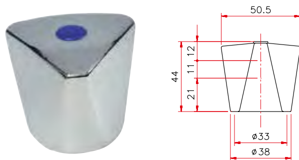
Art. 173 Maniglia Lena
