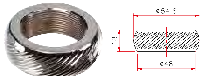
Art. 053 Anello Italia
