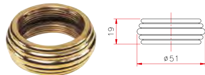
Art. 003 Anello America R.
