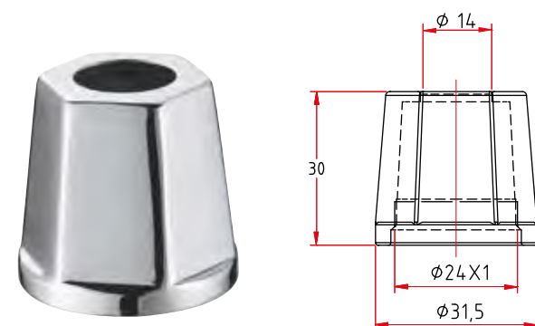
Art. 325 Coprivitone Astoria
