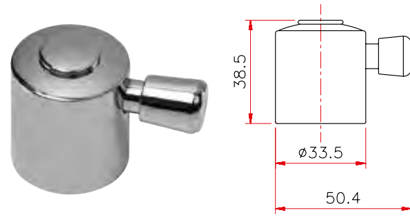
Art. 209 Deviatore Giuse
