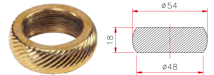
Art. 011 Anello Svizzera
