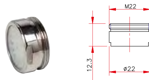
Art.453 Rompigetto maschio
