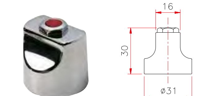
Art. 203 Deviatore Scricciolo
