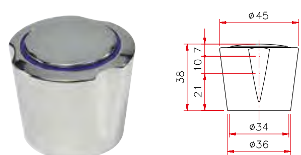
Art. 179 Maniglia Venere
