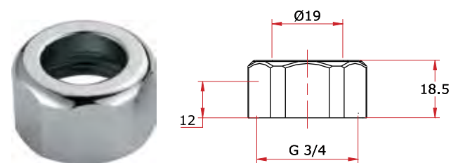
Art.445 Calotta Lusso
