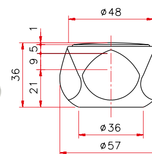
Art. 143 Maniglia Diamante
