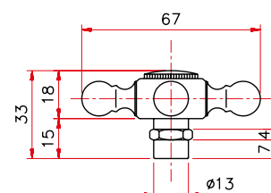
Art. 125 Maniglia Birillo Classico
