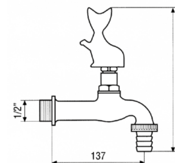
Art. 954 Rubinetto con maniglia delfino Robinet avec poignée à dauphin Tap with dolphin handle
