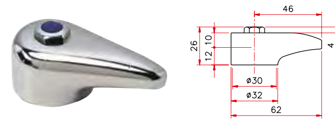
Art. 221 Deviatore Export
