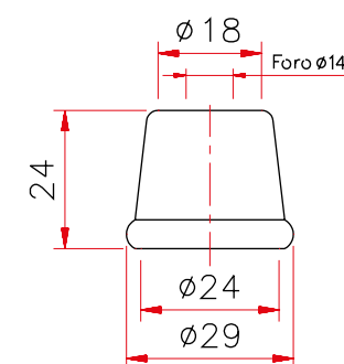
Art. 301 Coprivitone Tondo C
