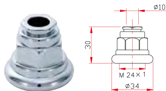
Art. 321 Coprivitone Retrò
