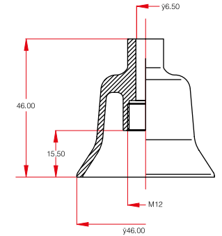
Art. 467 Cappuccio Centrale
