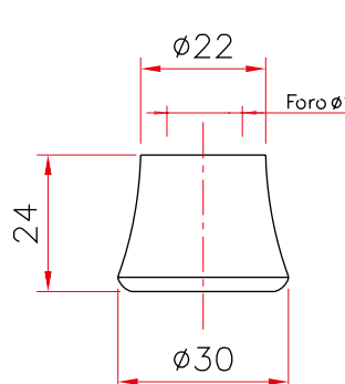
Art. 315 Coprivitone Classico R
