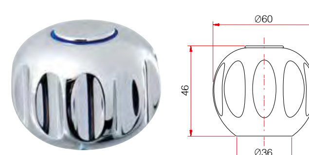
Art. 188 Maniglia Mandarino
