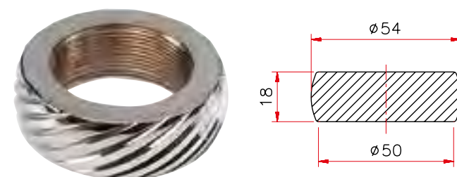
Art. 009 Anello Grecia
