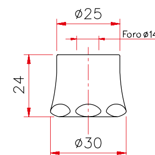
Art. 309 Coprivitone Esagono
