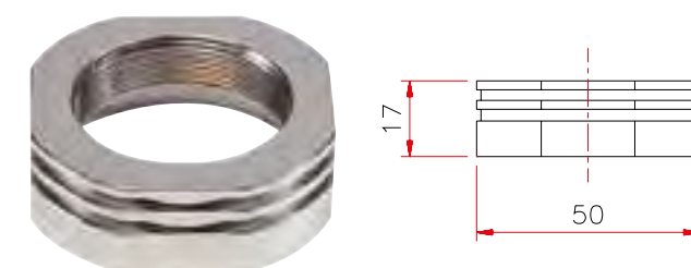
Art. 051 Anello Giappone
