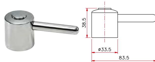
Art. 213 Deviatore Carmen
