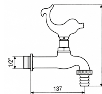
Art. 954 Rubinetto con maniglia delfino Robinet avec poignée à dauphin Tap with dolphin handle
