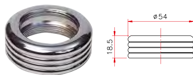
Art. 007 Anello Spagna
