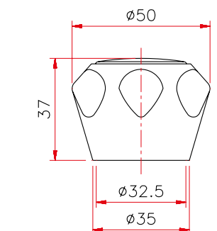
Art. 155 Maniglia Rubino
