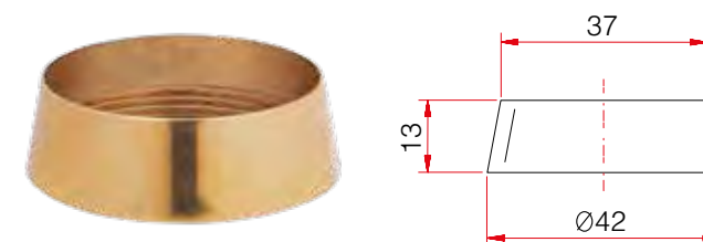
Art.452 Cappuccio Copricartuccia disponibile in varie dimensioni
