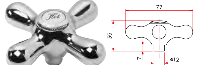
Art. 113 M. Fiocco Di Neve G.
