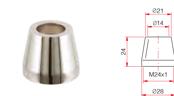
Art. 333 Coprivitone Egitto
