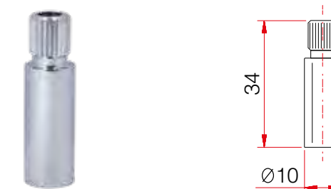
Art.689 Prolunga Broccia disponibile in varie dimensioni
