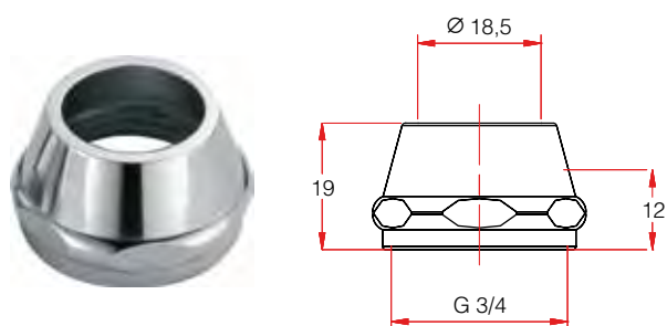
Art.449 Calotta Conica
