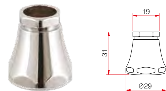
Art. 331 Coprivitone Martina
