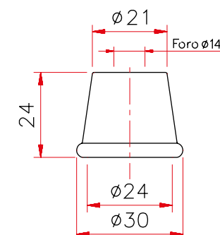
Art. 303 Coprivitone Tondo A
