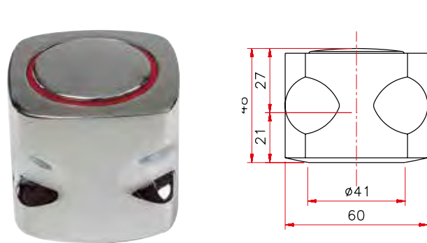
Art. 185 Maniglia Topazio/C
