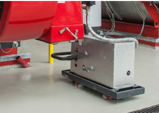
Ölzirkulationsmodul OCM
