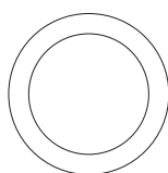
Art. STP01 - Ø 29 - (UT. Ø 21 - falda 4) Art. STP02 - Ø 31 - (UT. Ø 23 - falda 4) Art. STP03 - Ø 34,5 - (UT. Ø 25,5 - falda 4,5)
