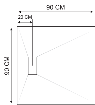
Piatto doccia 90 x 90
