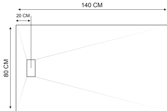
Piatto doccia 80 x 140
