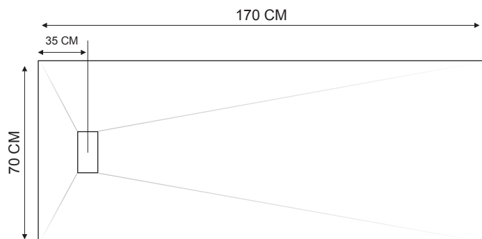
Piatto doccia 70 x 170
