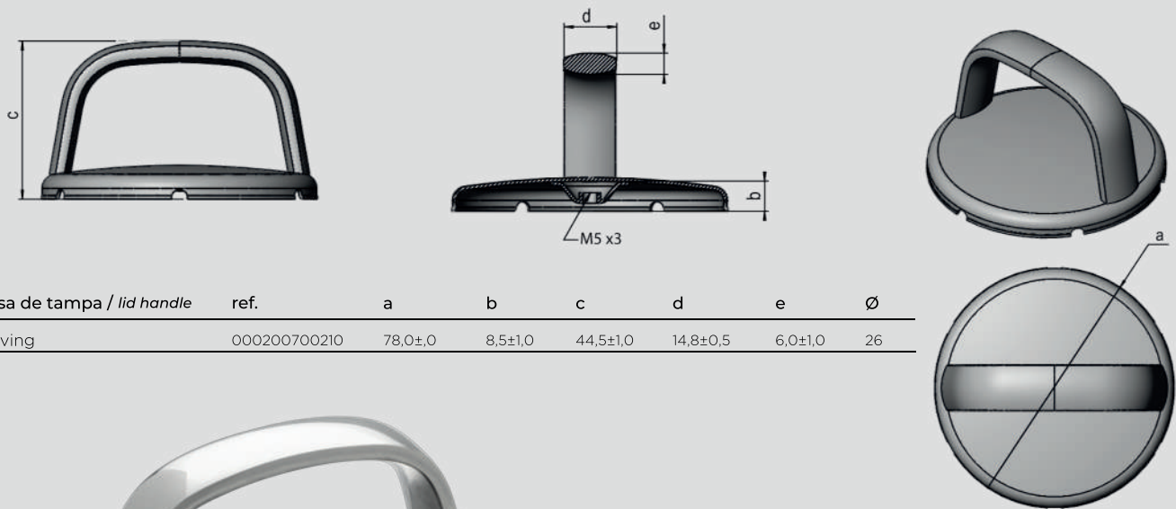
asa de tampa/ lid handle
