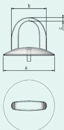
asa de tampa esmagada/ flat lid handle
