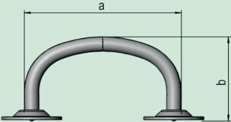
asa de tampa/ lid handle
