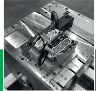
Spritzgusswerkzeuge
